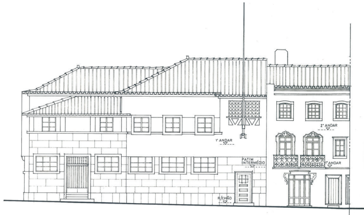
ALÇADO PRINCIPAL
