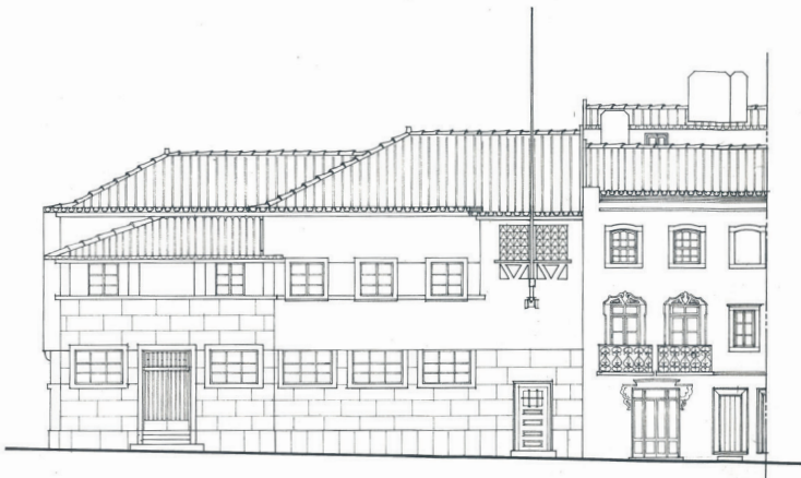
ALÇADO PRINCIPAL
